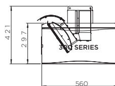
VOORPROFIEL (ZONDER WARMTE-AFLEIDER)
