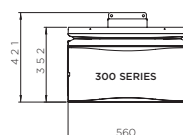
VOORAANZICHT (MET WARMTEREFLECTOR)
