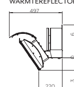
ZIJAAANZICHT (MET WARMTEREFLECTOR)
