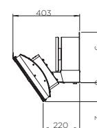
ZIJPROFIEL (ZONDER WARMTE-AFLEIDER)
