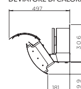
PROFILO LATERALE (CON DEVIATORE DI CALORE)
