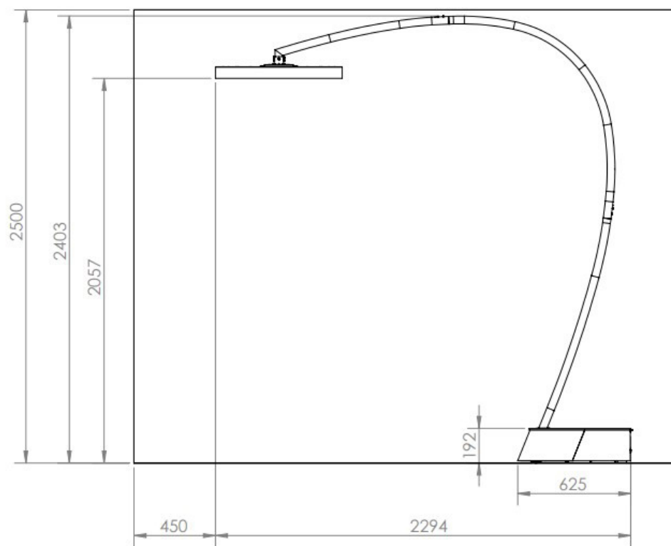
DÉGAGEMENT DU PLAFOND ET DES MURS
