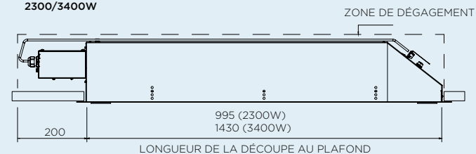
Trousse pour installation à faible dégagement au plafond 2300/3400W
