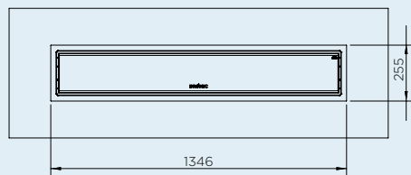
CAVITÉ MINIMUM FACULTATIF 2 2300/3400W
