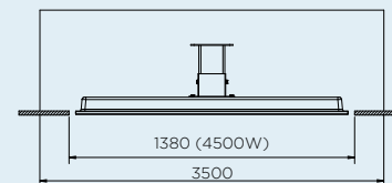
CAVITÉ MINIMUM 4500 W
