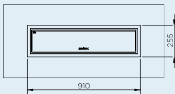
CHÂSSIS AFFLEURANT PLAFOND 2300 W
