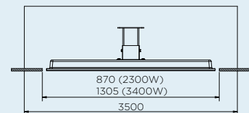
CAVITÉ MINIMUM FACULTATIF 2 2300/3400W
