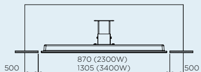
CAVITÉ MINIMUM FACULTATIF 1 2300/3400W
