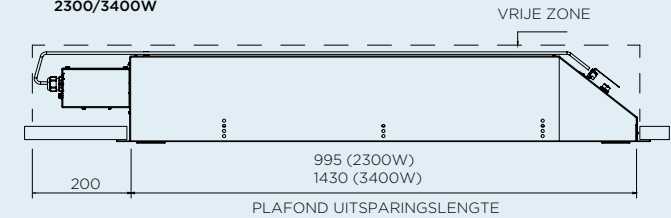
UITSPARINGSKIT VOOR WEINIG VRIJE RUIMTE 2300/3400W
