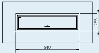
PLAFONDINBOUWFRAME 2300W
