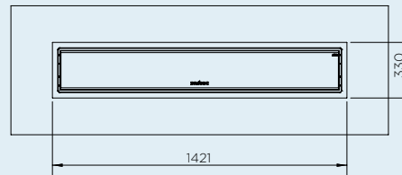
MINIMALE INBOUWRUIMTE 4500W
