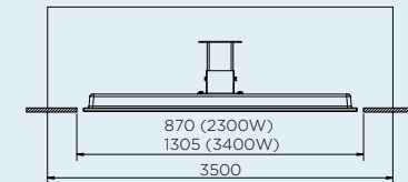
MINIMALE INBOUWRUIMTE OPTIE 2 2300/3400W
