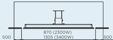
MINIMALE INBOUWRUIMTE OPTIE 1 2300/3400W
