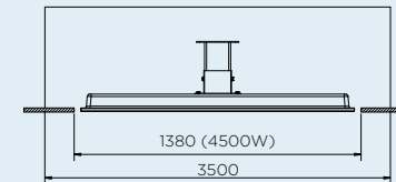
MINIMALE INBOUWRUIMTE 4500W
