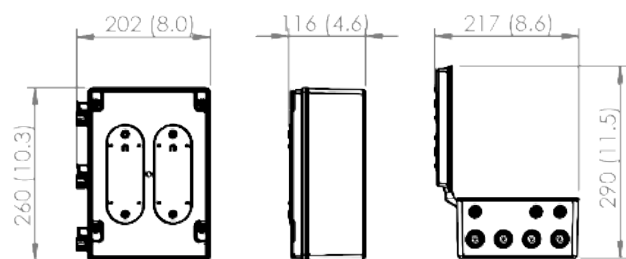
Afmetingen weergegeven in mm (inches)
