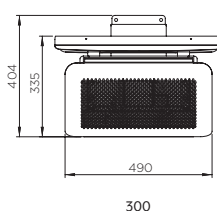
VOORZICHT (MET WARMTEDEFLECTOR)
