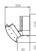
ZIJPROFIEL (ZONDER WARMTE-AFLEIDER)
