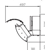
ZIJPROFIEL (MET WARMTE-AFLEIDER)
