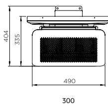
VUE DE FACE (AVEC DÉFLECTEUR DE CHALEUR)
