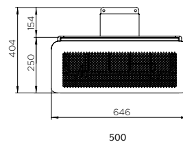
VUE DE FACE (AVEC DÉFLECTEUR DE CHALEUR)
