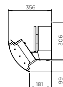
VUE DE FACE (SANS DÉFLECTEUR DE CHALEUR)
