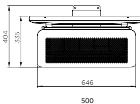
VUE DE FACE (AVEC DÉFLECTEUR DE CHALEUR)
