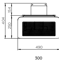
VUE DE FACE (AVEC DÉFLECTEUR DE CHALEUR)
