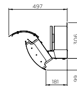
VUE DE FACE (SANS DÉFLECTEUR DE CHALEUR)
