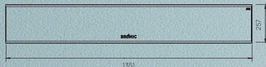
Dimensions 4500W :
