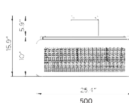
VUE AVANT (SANS DÉFLECTEUR DE CHALEUR)
