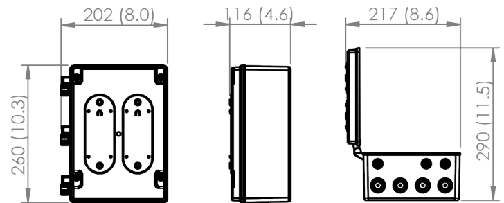
DISPOSITIVO ON/OFF DE 1 Y 2 CANALES
