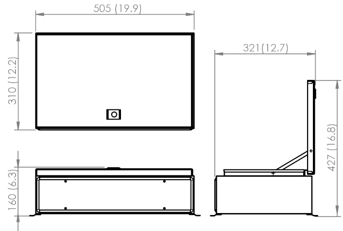
DISPOSITIVO ON/OFF DE 5 CANALES
