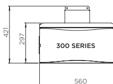
FRONTANSICHT (OHNE WÄRMESCHUTZ)
