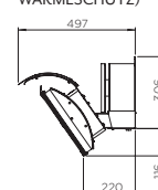
SEITENANSICHT (MIT WÄRMESCHUTZ)
