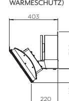
SEITENANSICHT (OHNE WÄRMESCHUTZ)
